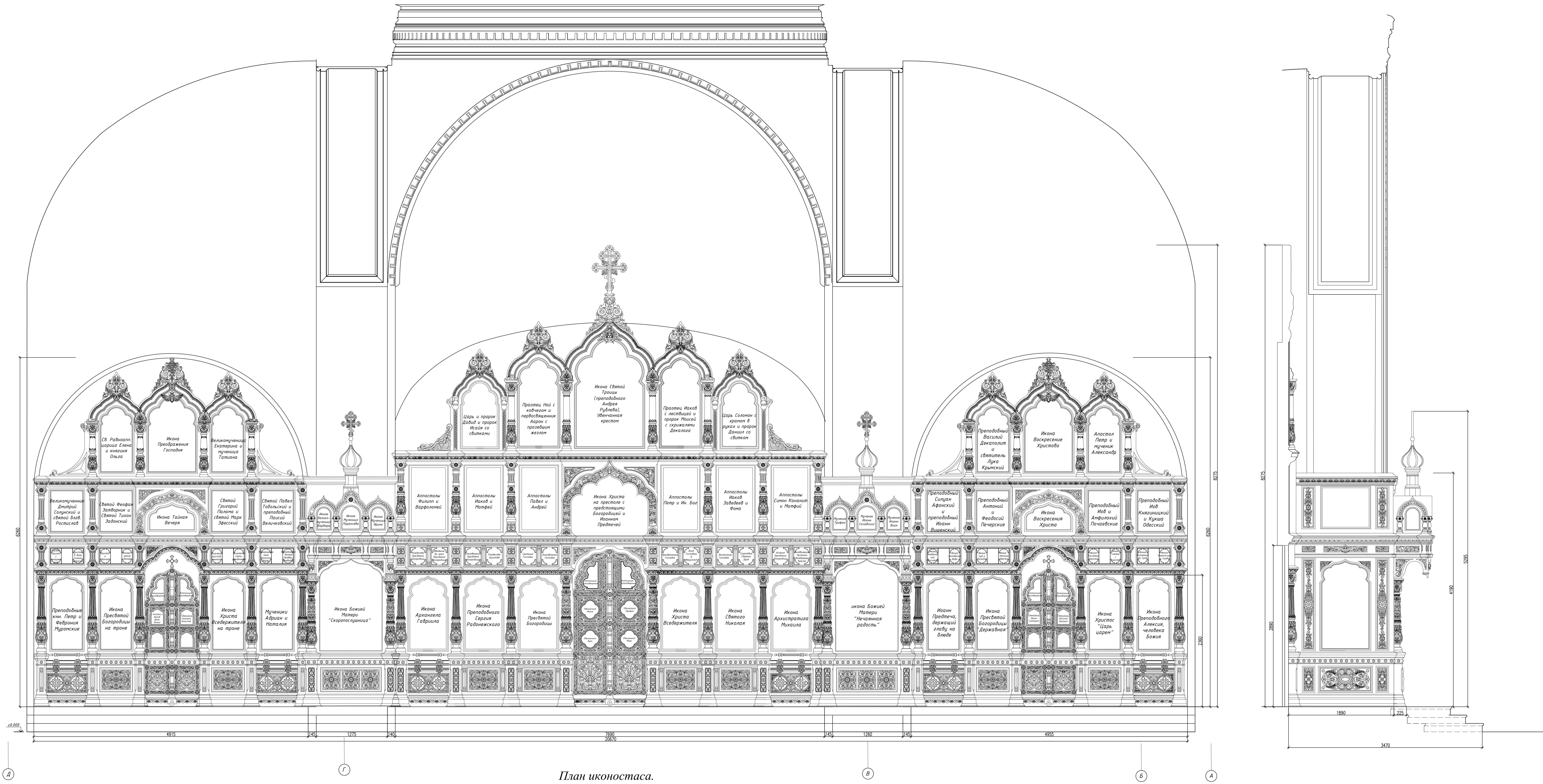
Иконостас. Фасад. Масштаб 1:25
